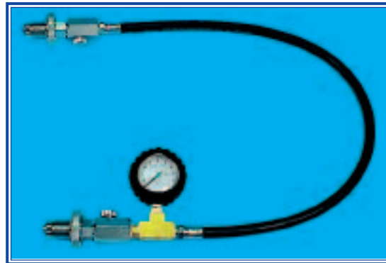
A136 DIN Tank to DIN tank equalizer with 5000 psi gauge
