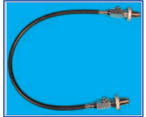
A134 DIN Tank to DIN tank equalizer line with bleeder
